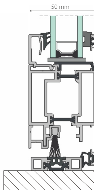
PRZEKRÓJ PRZEZ DRZWI PI 50N
